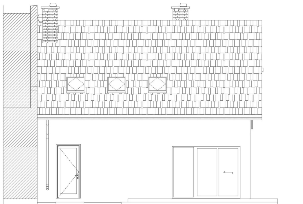
ELEWACJA POŁUDNIOWA
