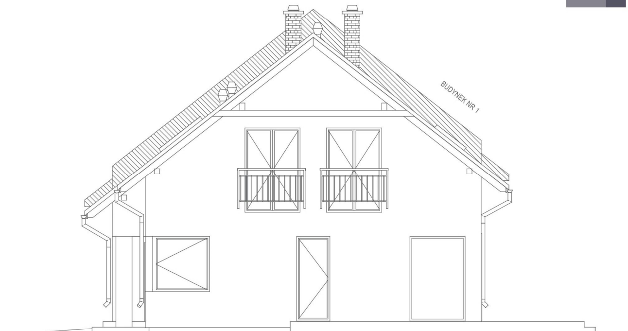
ELEWACJA WSCHODNIA
