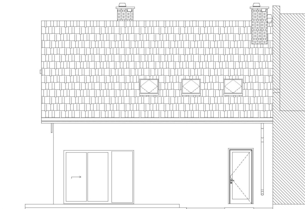
ELEWACJA POŁUDNIOWA
