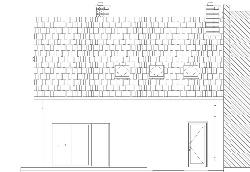
ELEWACJA POŁUDNIOWA
