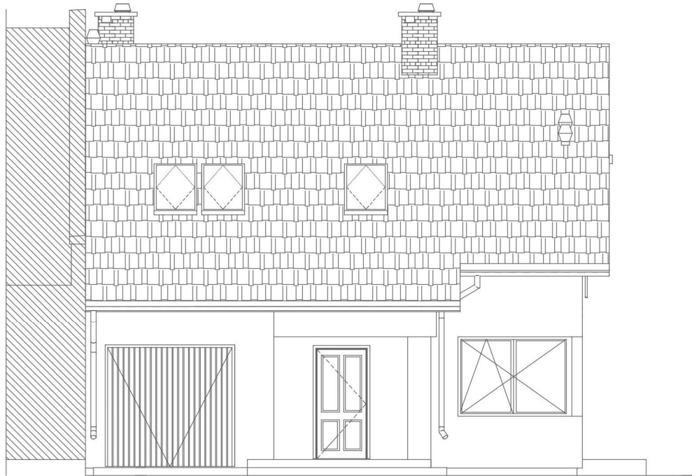
ELEWACJA PÓŁNOCNA
